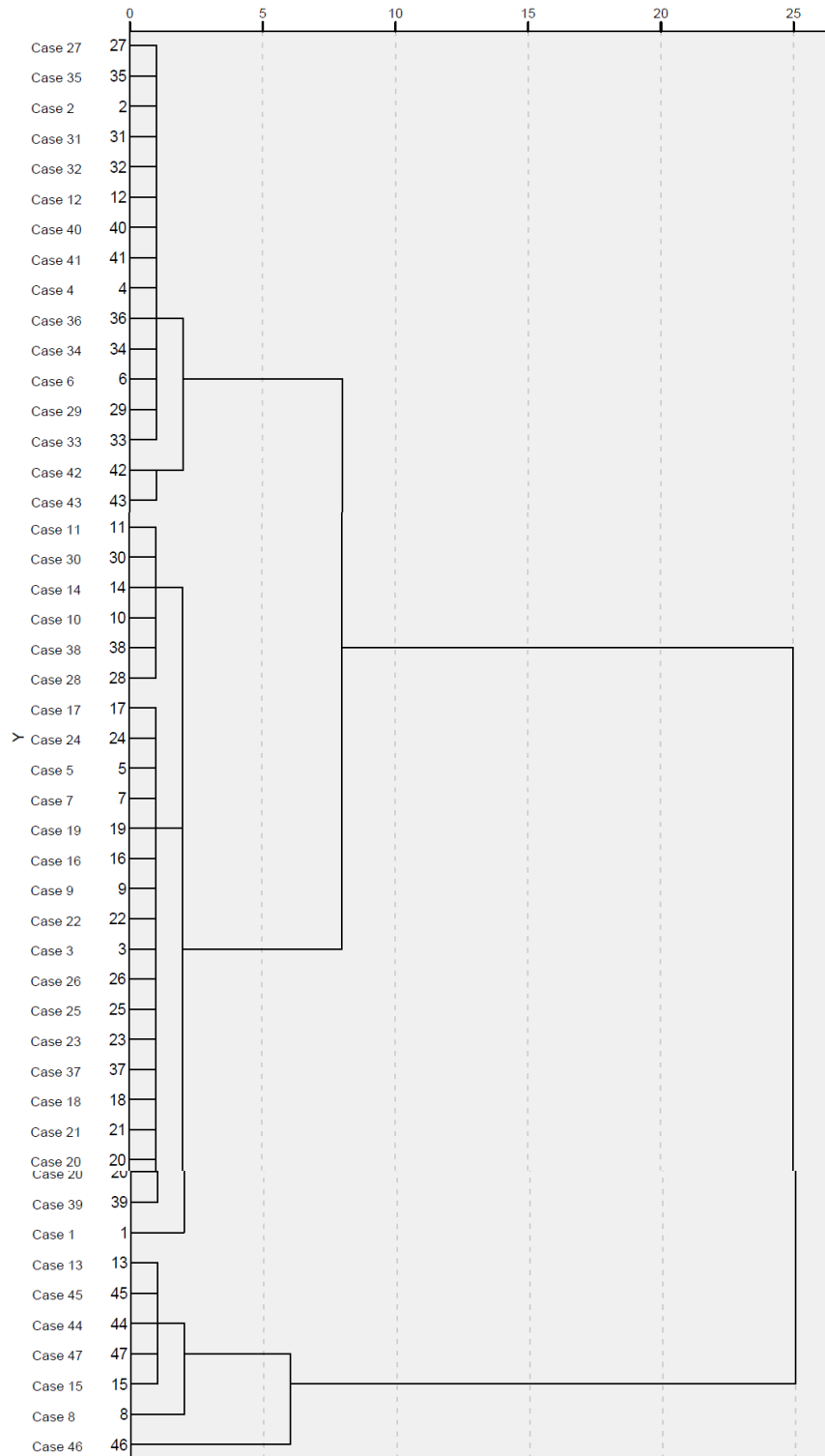
Figura 35. Dendrograma que utiliza un enlace Ward, combinación de clúster de sustancias re-escalada.
