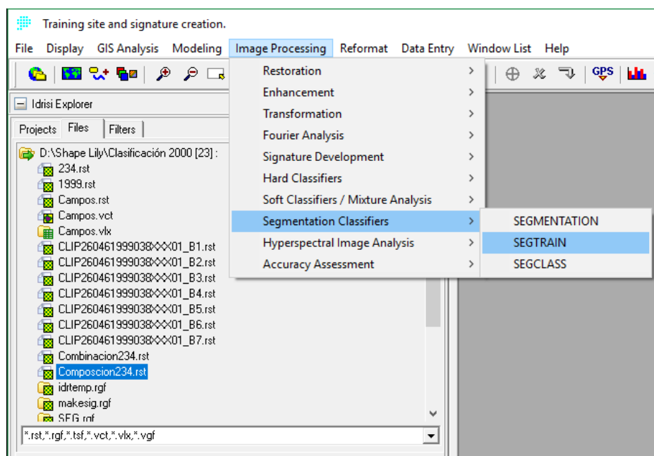
Figura 9. Herramienta SEGTRAIN.
