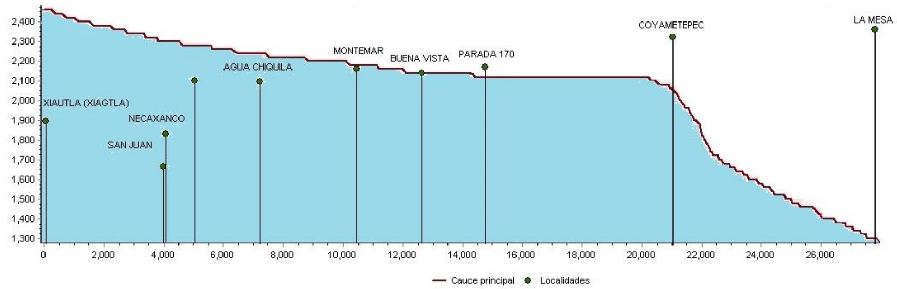
Figura 28. Perfil longitudinal del cauce de la microcuenca 17, Acaxochitlán, Hidalgo.
