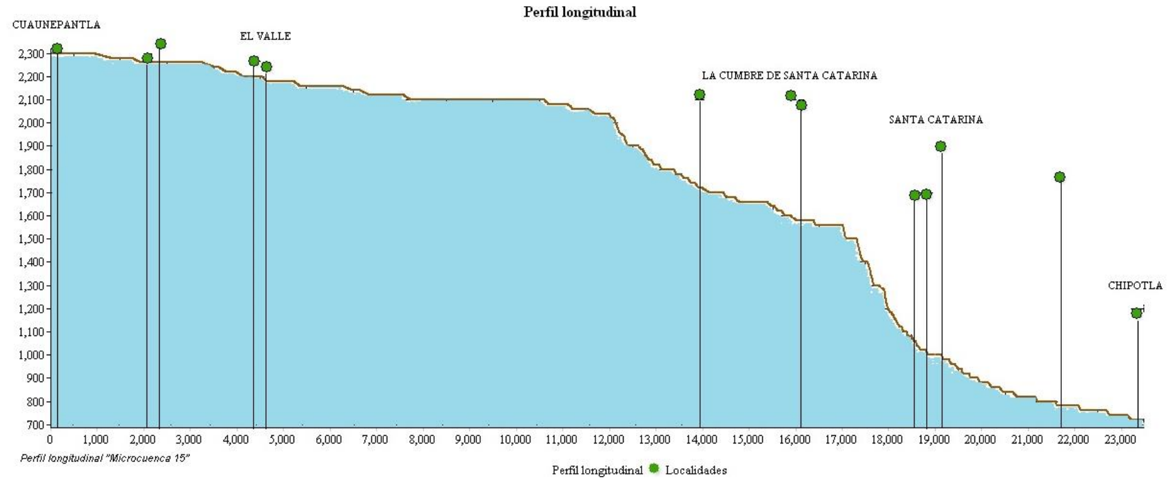
Figura 27. Perfil longitudinal de la microcuenca 16, Acaxochitlán, Hidalgo.
